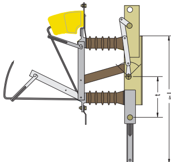
Bauform H 22 EA mit unten angebautem Erdungsschalter
