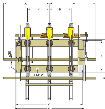
Bauform H 22 EA mit unten angebautem Erdungsschalter
