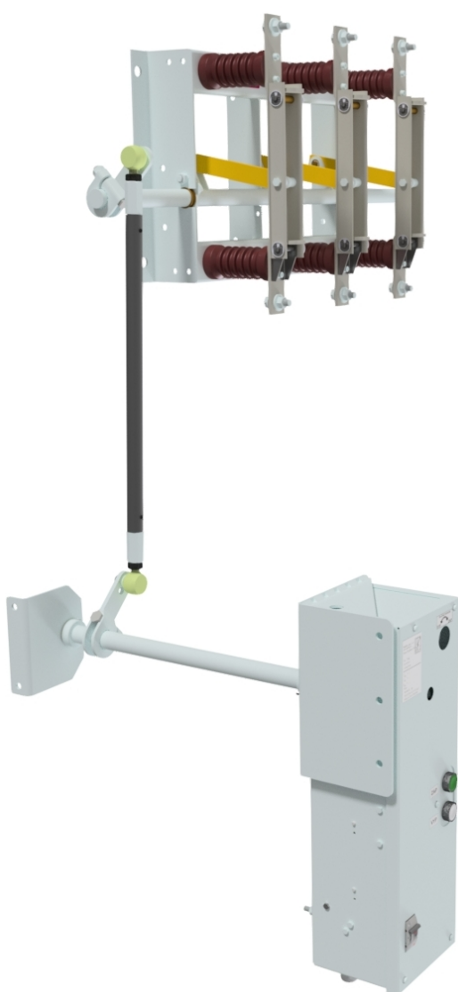
Pohon VM20, DT montovaný vlevo – zapnutý stav
